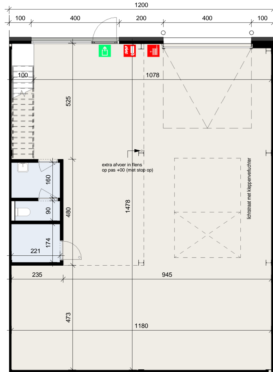
Gelijkvloers 1 : 100
